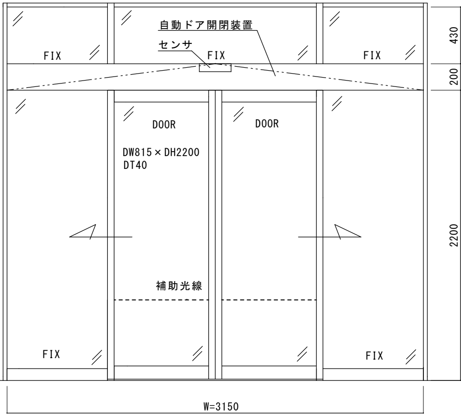
内観図
