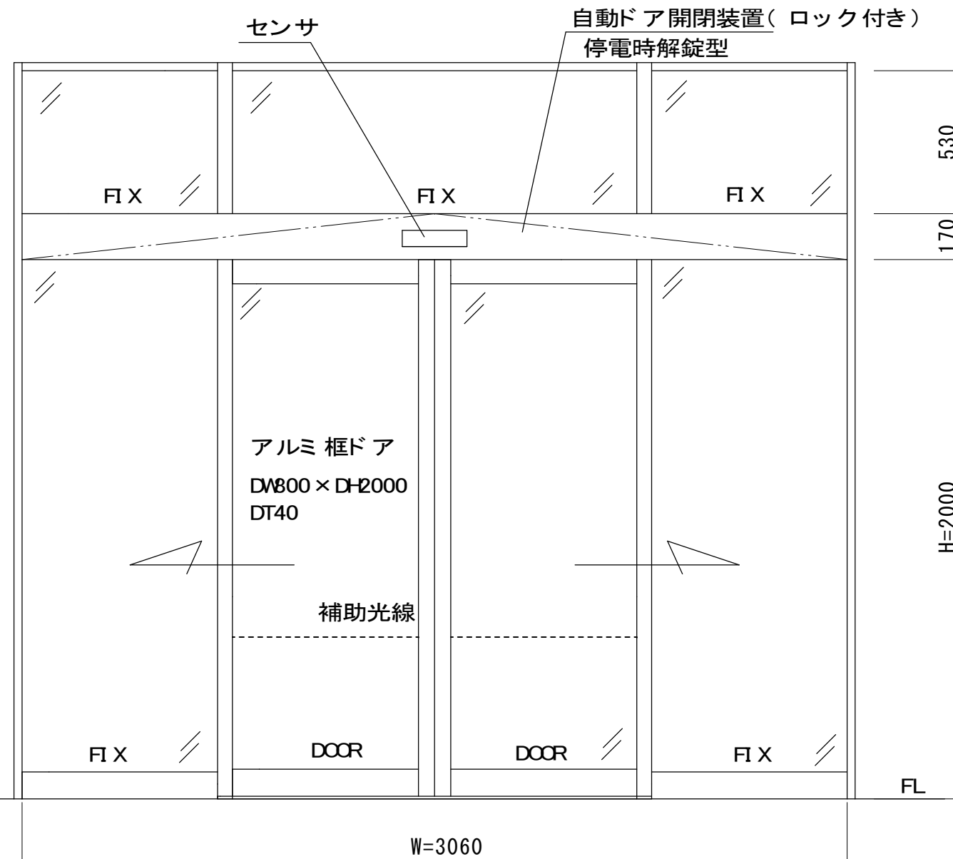
内観図
