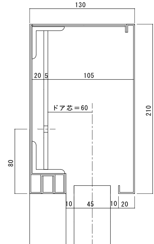
無目断面詳細図
