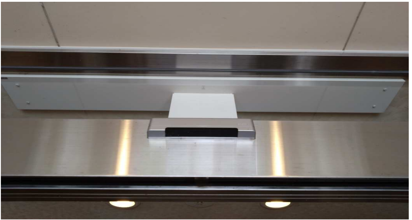
内側起動センサ（無目付けセンサ）
