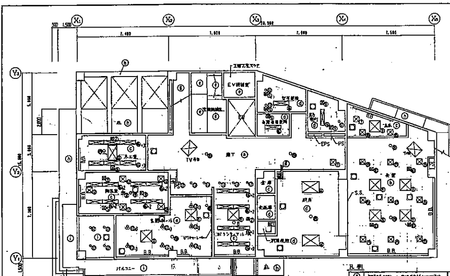
1階 天井伏図 S1:100
