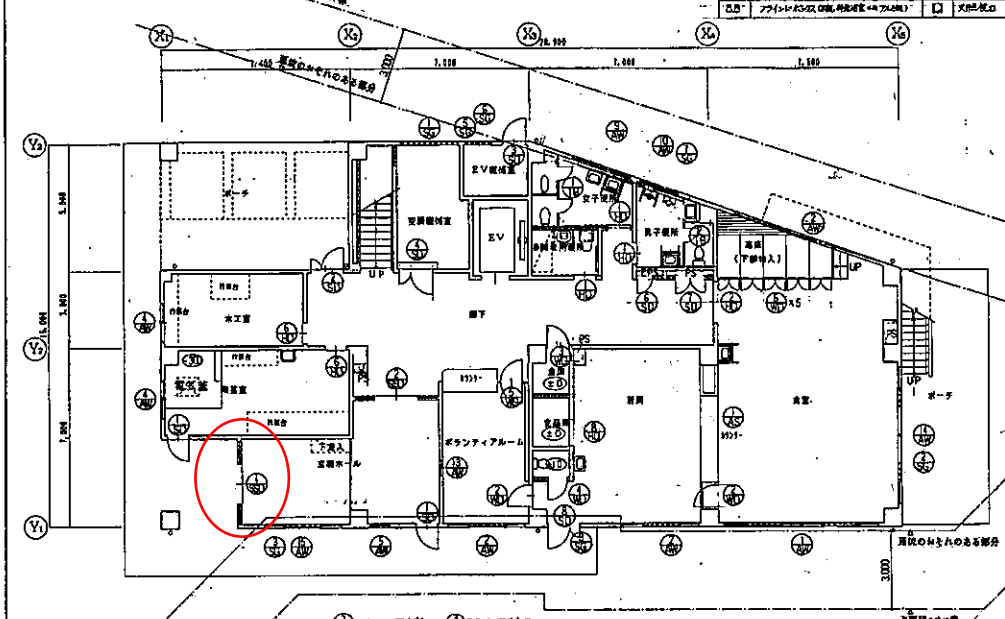
1階 建具案内図 S1:100
