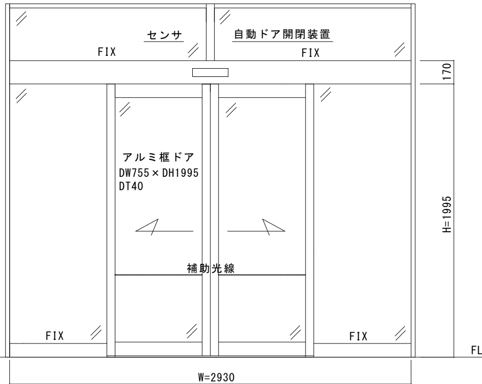
内観図
