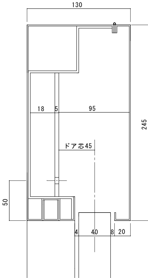
無目断面詳細図
