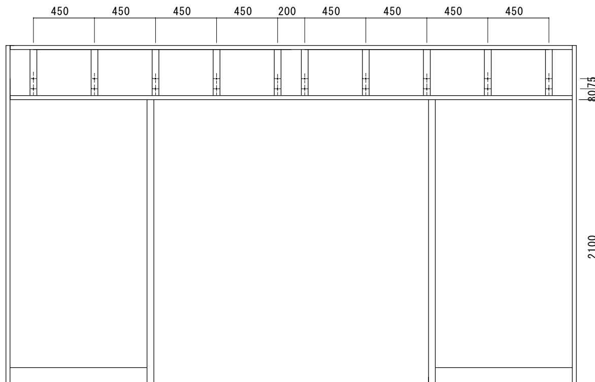
FB割付図
