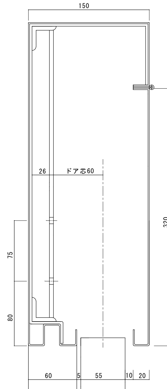
無目縦断面詳細図
