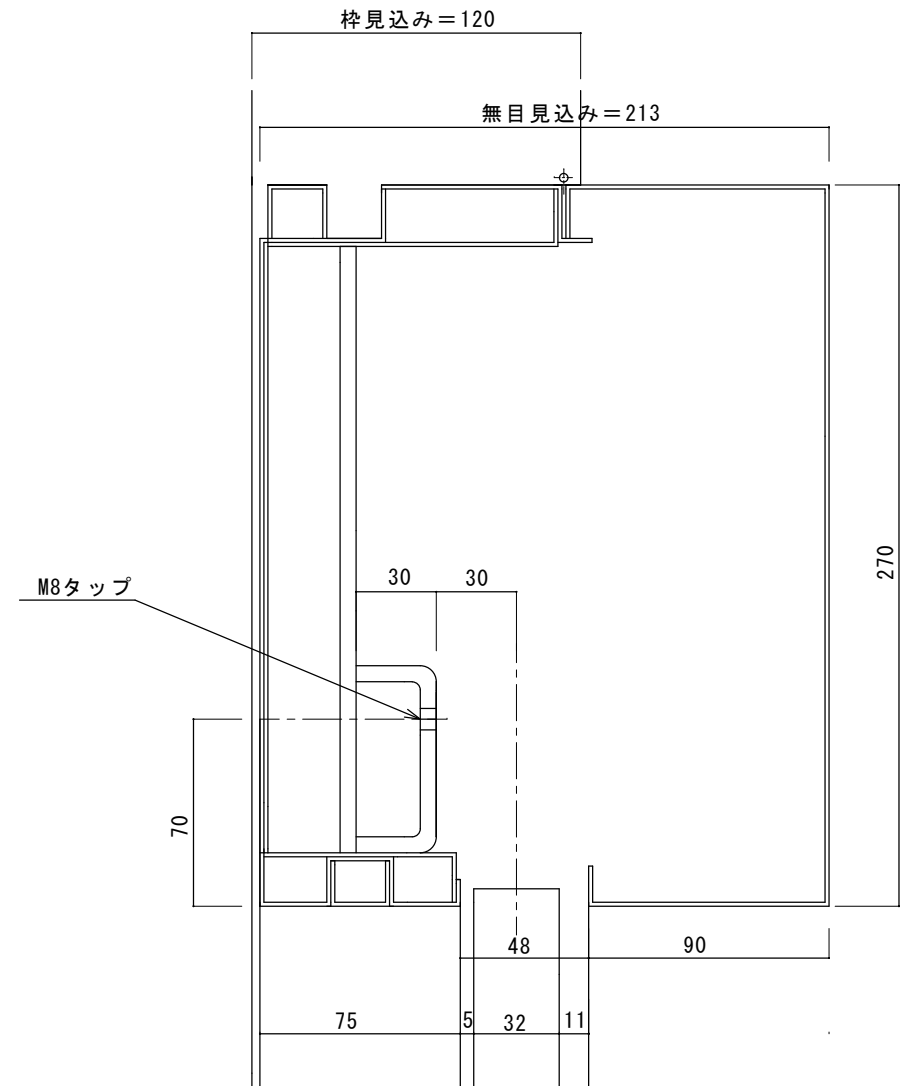
無目断面詳細図
